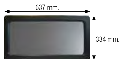
Ventana con metacrilato. Dimensiones: 550 x 245 mm.
