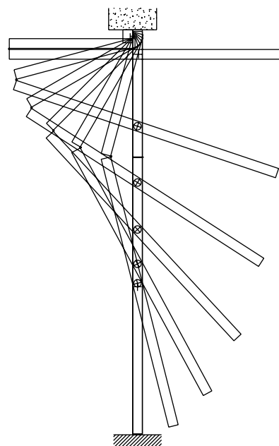
FIGURA 2 Detalle de apertura de puerta industrial basculante
