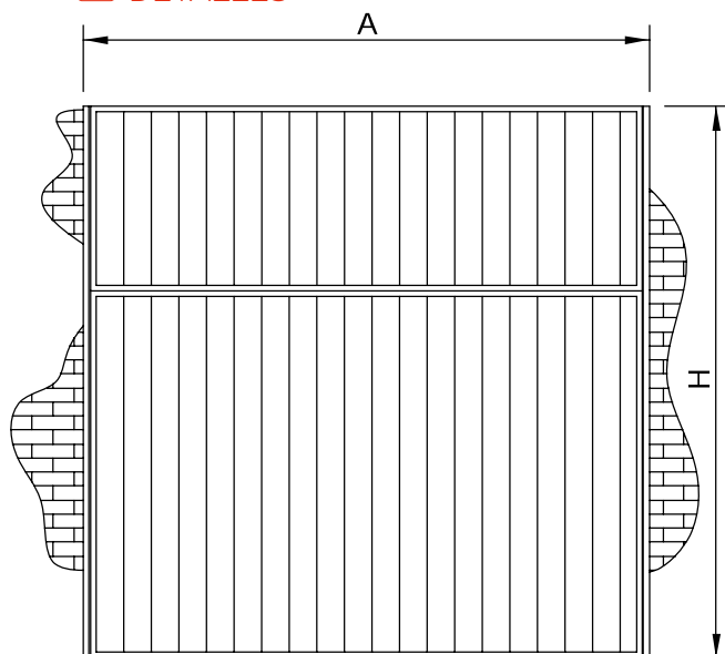
FIGURA 1 Detalle de alzado de puerta industrial basculante
