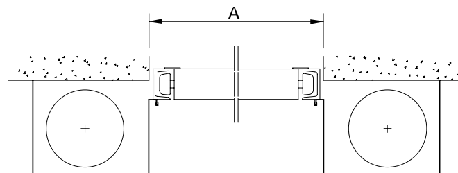
FIGURA 4. Detalle de planta de puerta industrial basculante con contrapesos ocultos protegidos con forros
