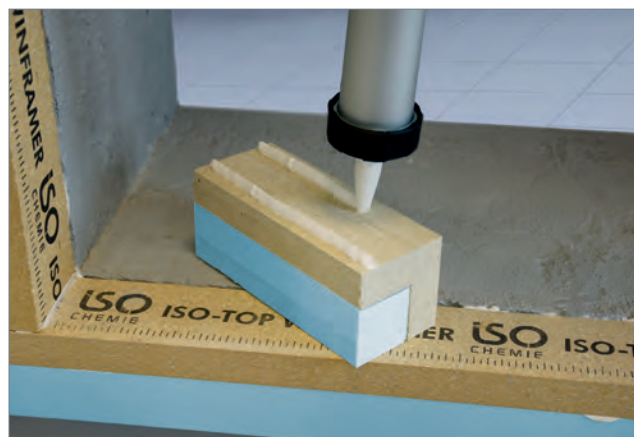
Ejemplo de instalación: ISO-TOP FLEX-ADHESIVE WF
