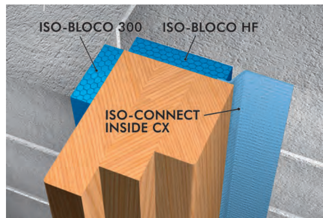
Ejemplo de instalación: SISTEMA DE SELLADO DE VENTANAS ISO 3
