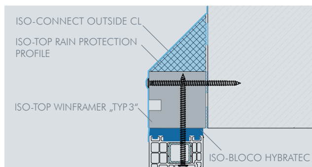
Ejemplo de instalación: ISO-TOP RAIN PROTECTION PROFILE
