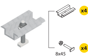
Grapa intermedia con tornillo
