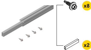
Conector con tornillos
