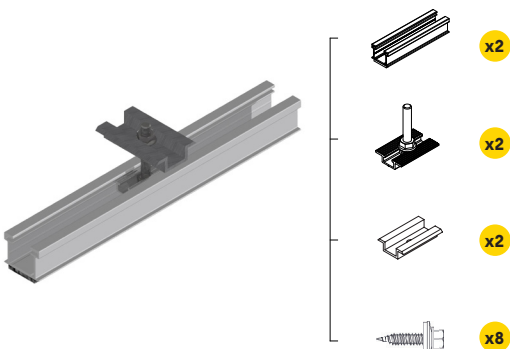
Tramo de perfil 300 mm con grapa intermedia
