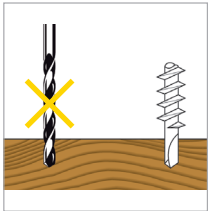
Fácil inicio del taladro. Para evitar un pretaladro en el montaje
