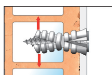
Taco fijado con doble expansión
