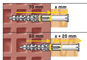
MFR 10: Ahora con doble empotramiento.
