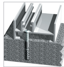
Taco en pared:
