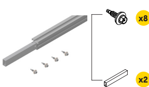
Conector con tornillos
