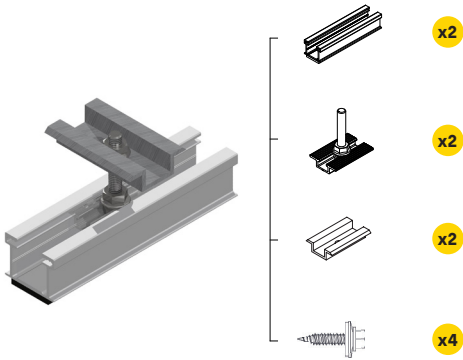
Tramo de perfil 150 mm con grapa intermedia
