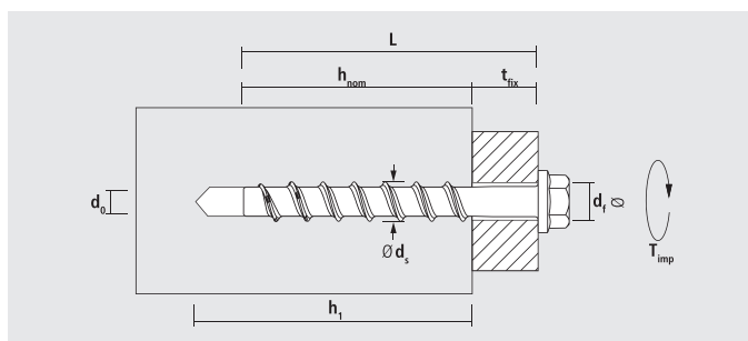
Montaje BTS 6 B
