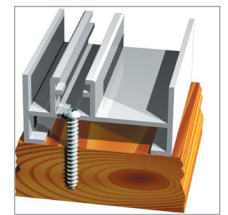
Premarco de madera:
